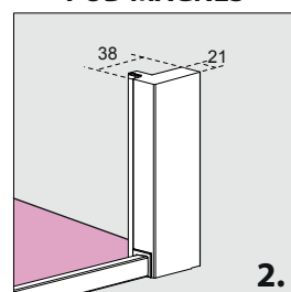
PROFIL PRZYŚCIENNY POD MAGNES
