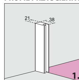
PROFIL PRZYŚCIENNY
