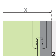
WYMIARY DO ZEWNĘTRZNEGO OBRYSU PROFILU
