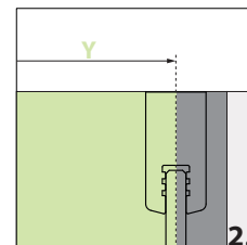
WYMIARY DO OSI/ŚRODKA SZYBY
